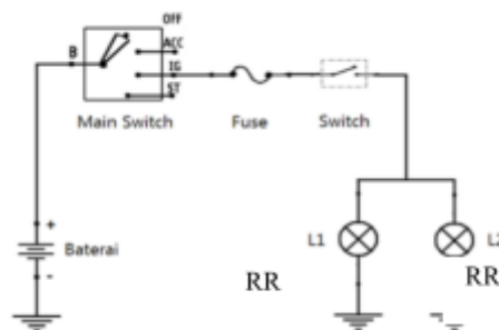
Gambar 1. Rangkaian Lampu Mundur
