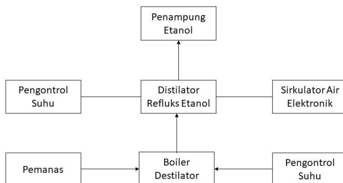
Gambar 1.(Bold, 10 pt, Times NewRoman) Diagram proses pembuatan bioetanol dengan teknik refluks (Tidak bold, 10 pt, Times New Roman)
