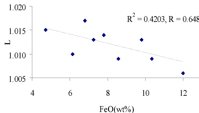
Gambar 1. Plot Lineasi (L) dan Kandungan FeO Menunjukkan Korelasi Negatif
