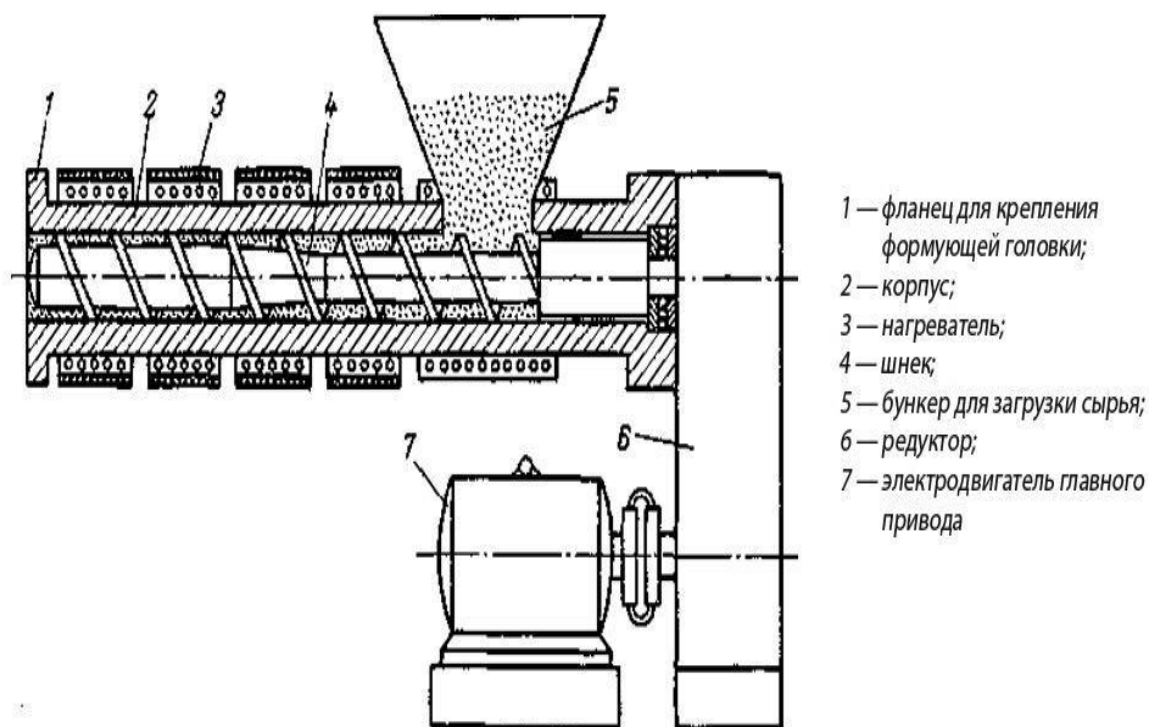
РИС. 1 СХЕМА ОДНОШНЕКОВОГО ЭКСТРУДЕРА
