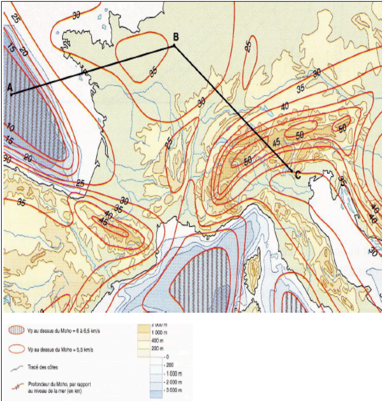
Carte topographique de l'Europe sur laquelle ont été placées les profondeurs du Moho en km
