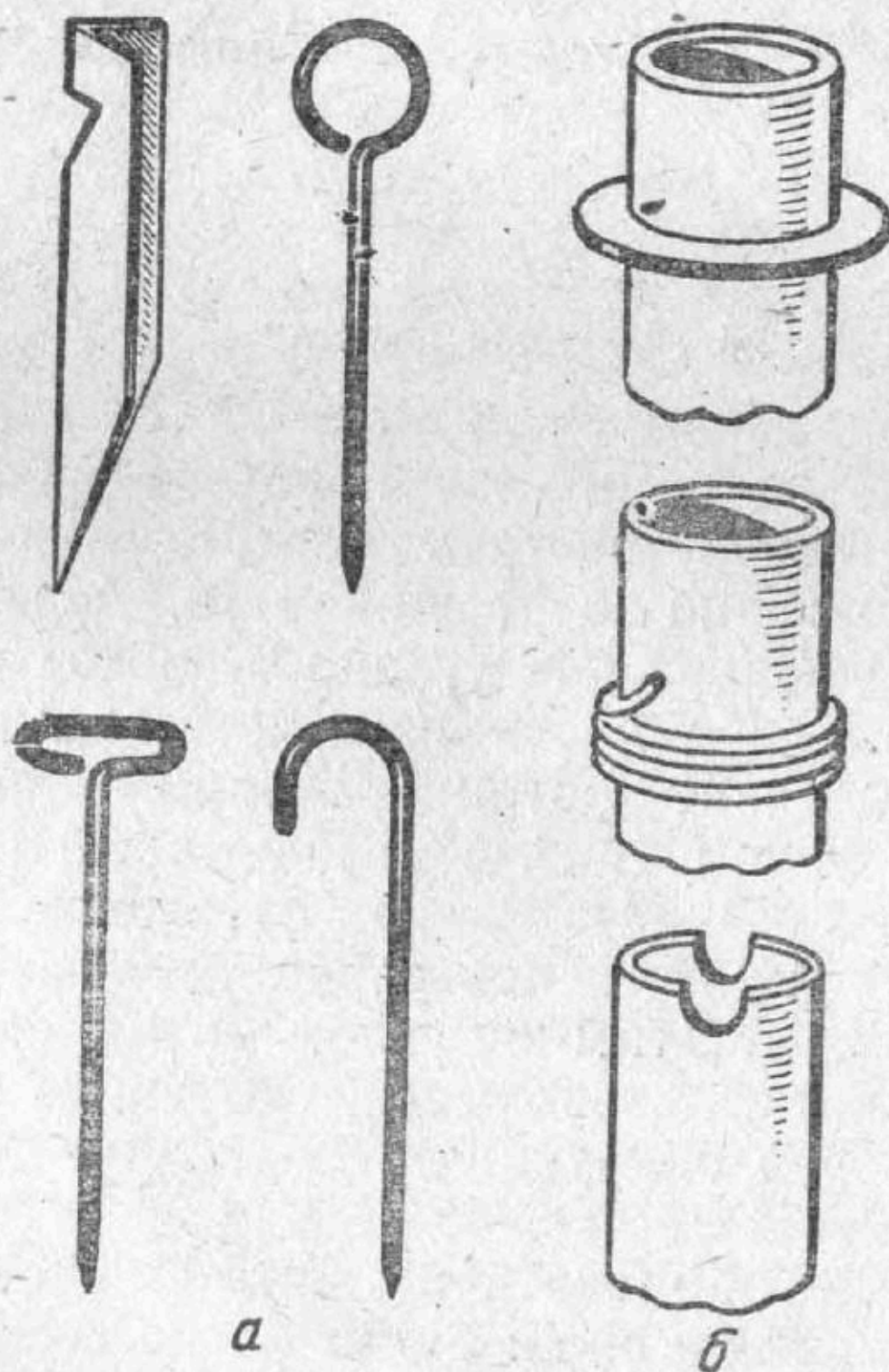
Рис. 19. Металлические штыри и опорные стойки для палатки.
