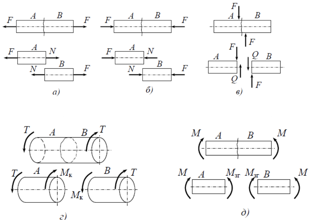
Рисунок 3. – Види деформації стержня:
