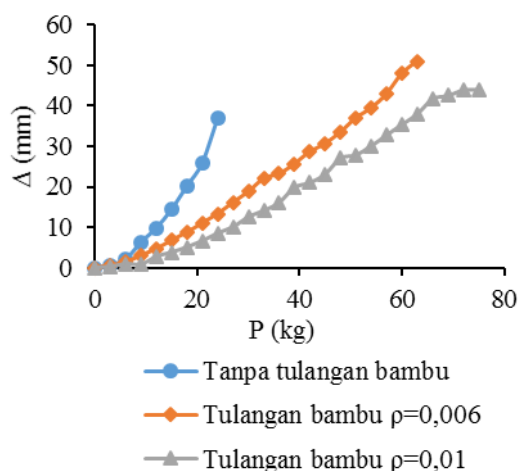
Gambar 1. Grafik hubungan P-Δ (Model A)
