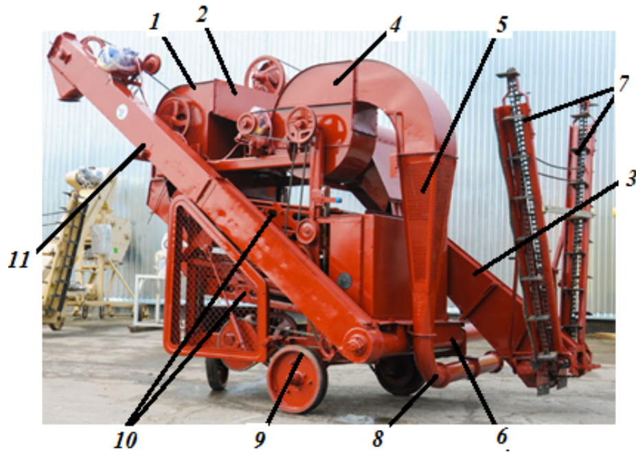
Рис. 10.1. Будова очисника вороху ОВС-25:
