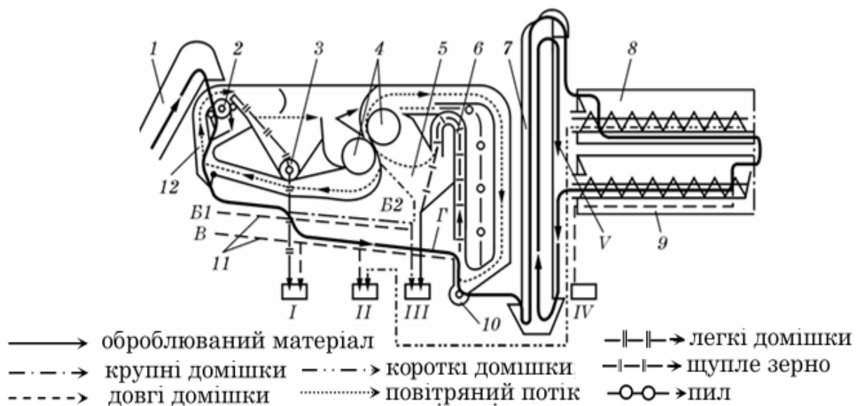
Рис. 10.5. Функціональна схема насіннеочисної машини СМ-4А:
