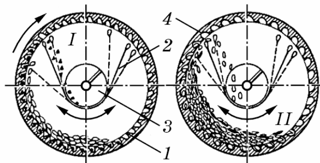
Рис. 10.6. Схема роботи трієрних циліндрів насіннеочисної машини СМ-4А:
