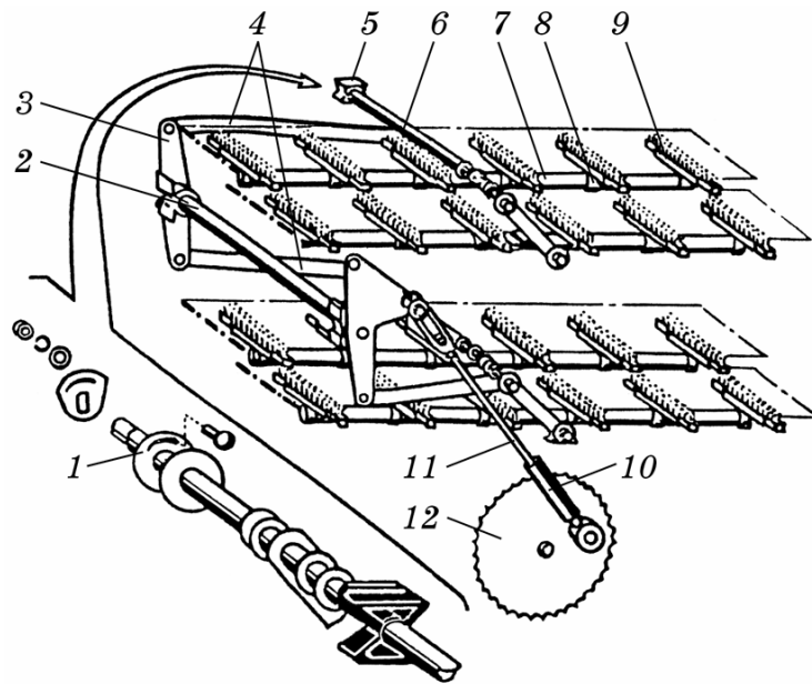
Рис. 10.2. Механізм очищення решіт ОВС -25:
