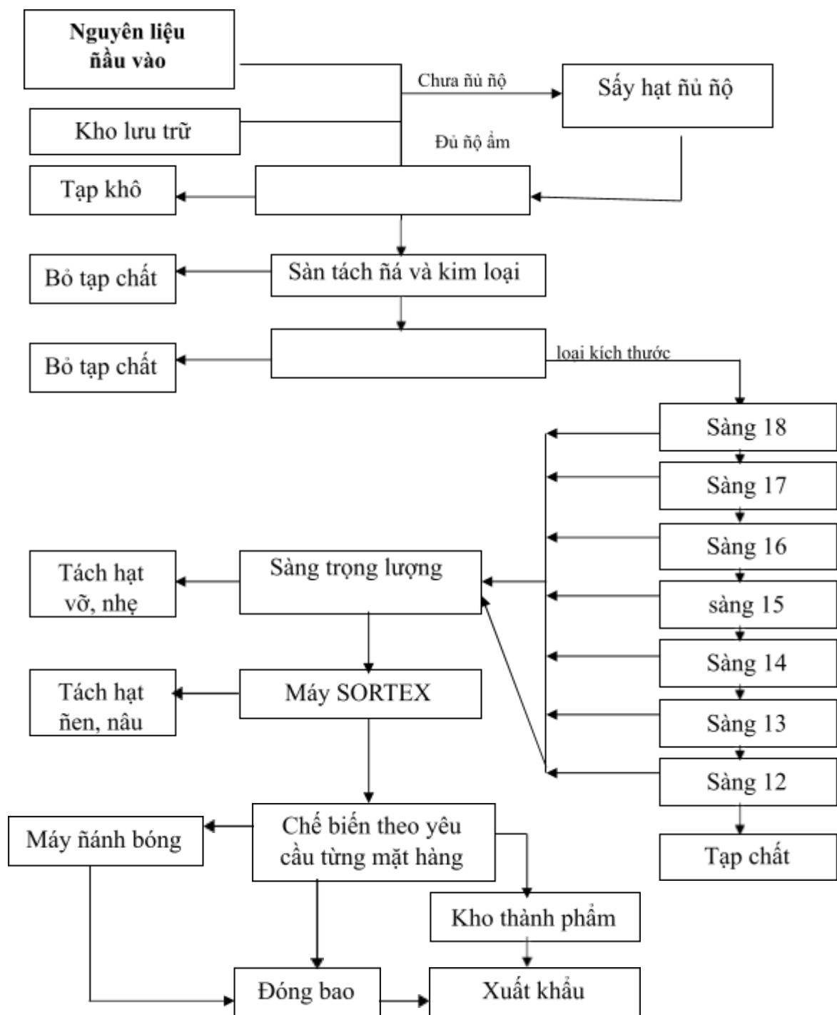
Sơ nũ 2.4 Đảm bảo chất lượng trong khâu sản xuất
