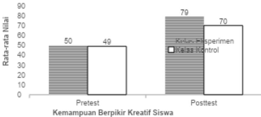
Gambar 1. Hasil Peningkatan Kemampuan Berpikir Kreatif Siswa
