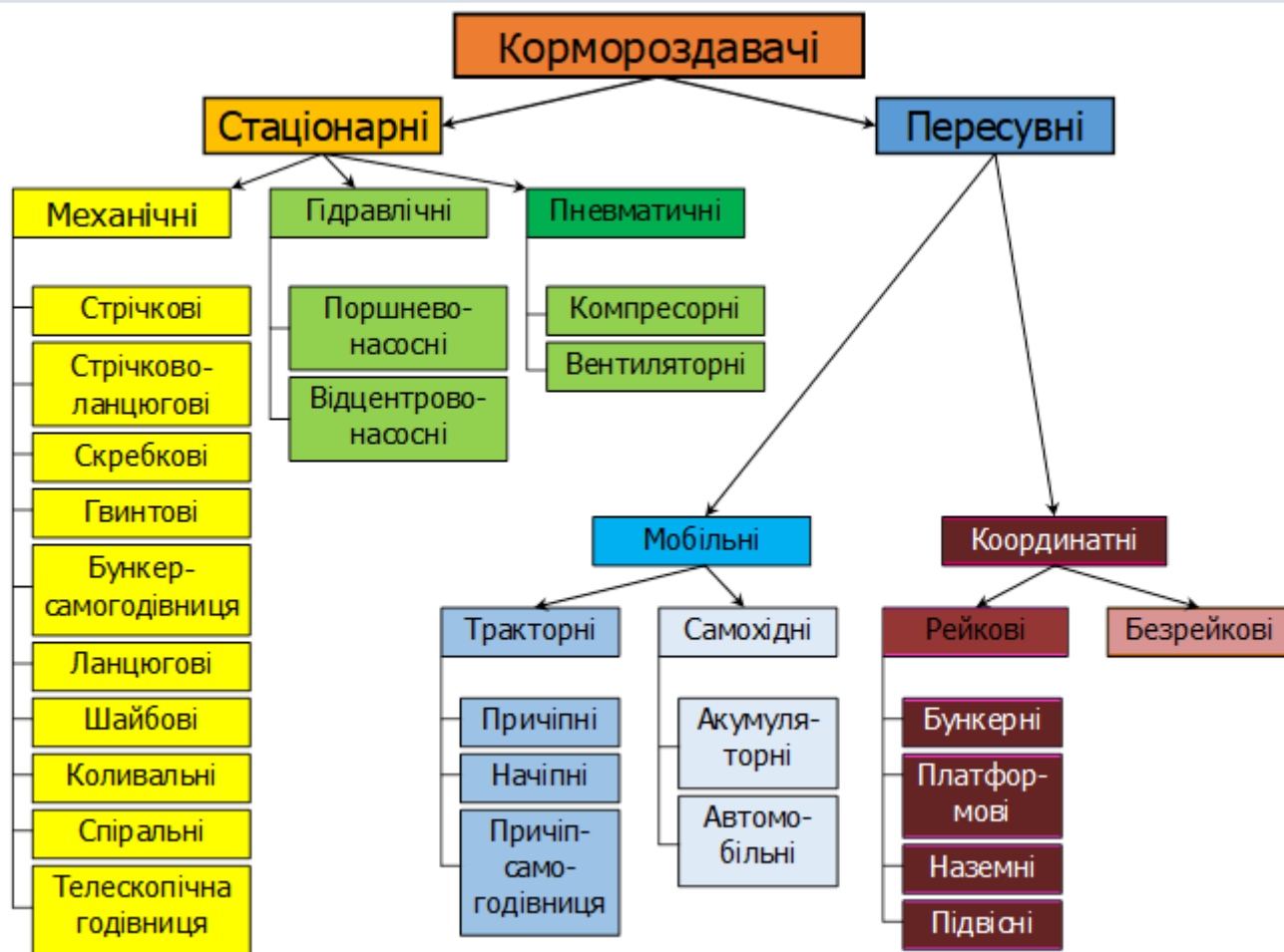
Рис. 5.1. Класифікація кормороздавачів
