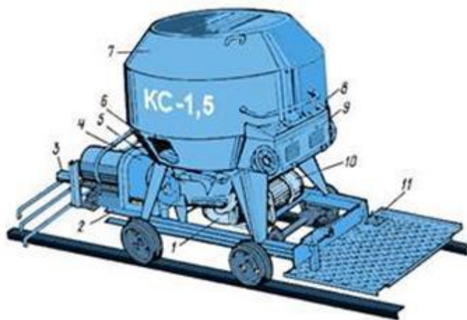
Рис. 5.12. Кормороздавач-змішувач KC-1,5:
