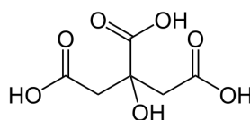
acide citrique
