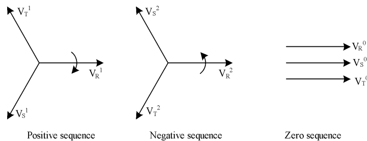
Gambar 1. Urutan Phasor Lengkap
