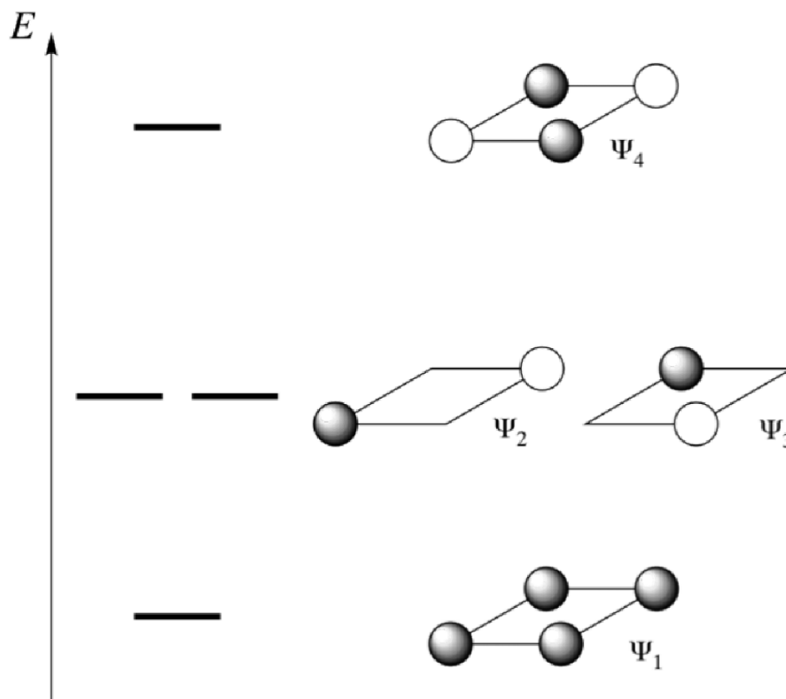
Figure 3 Orbitales d'un fragment « plan carré » X_4
