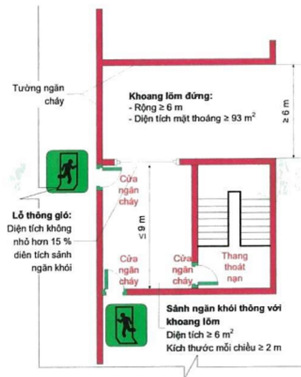
e) Khoảng đệm không nhiễm khói là một sảnh có thông gió tự nhiên với khoảng đệm
