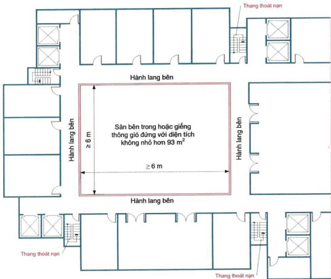
k) Khoảng đệm không nhiễm khói đi theo hành lang bên
