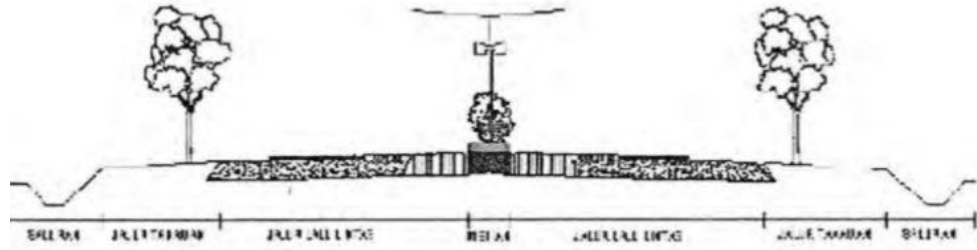
Gambar 3.1 Contoh tata letak jalur hijau jalan Sumber: http://www.penataanruang.net/itaru/upload/nspk/pedoman/R TH/7. (2006)
