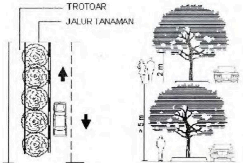
Gambar 3.2 Jalur tanaman tepi peneduh Sumber: http://www.penataanruang.net/itaru/upload/nspk/pedoman/R TH/7. (2006)
