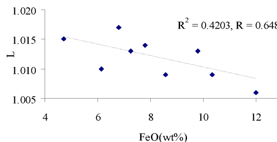
Gambar 1. Grafik garis (L) dan kandungan FeO yang menunjukkan korelasi negatif.
