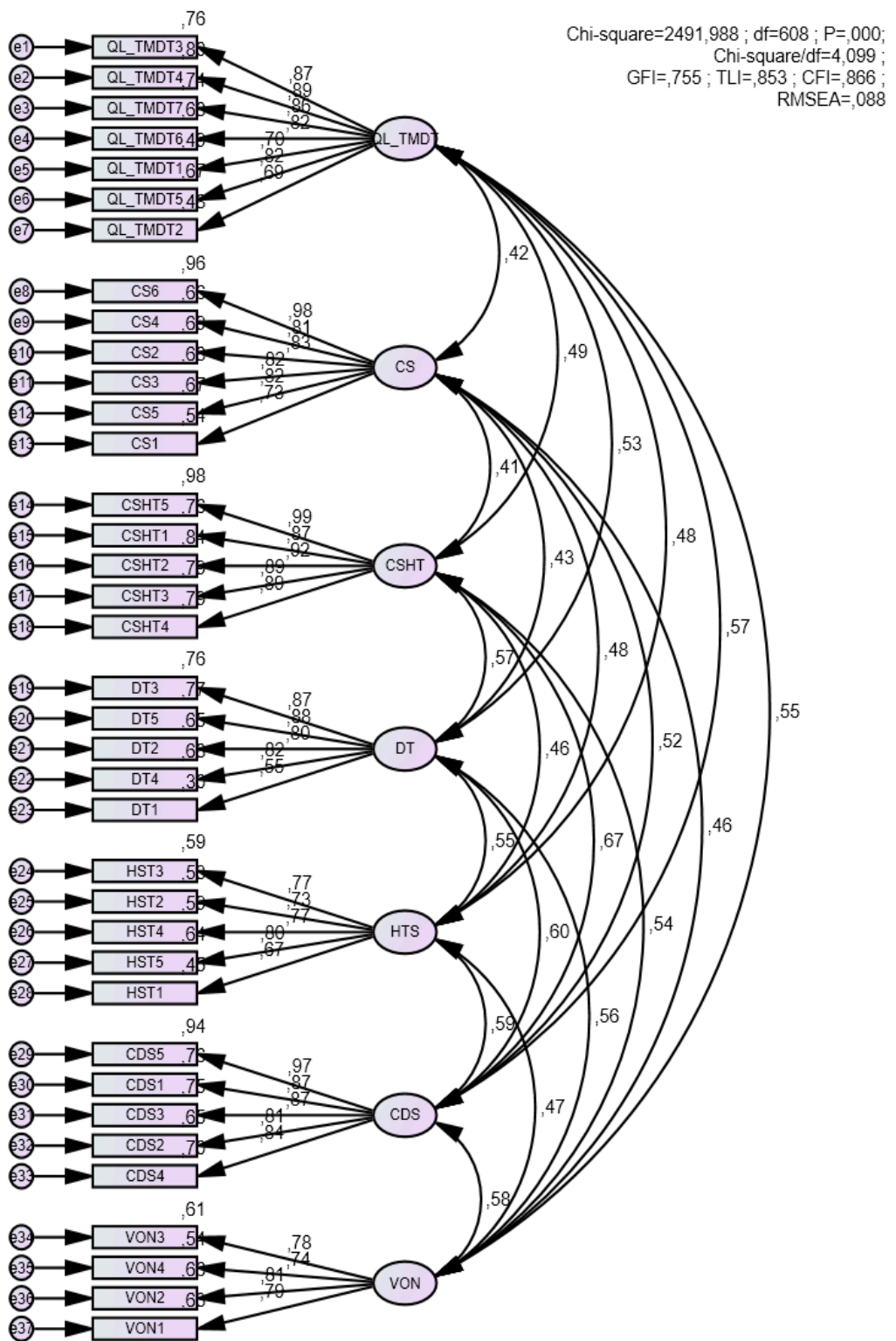
Hình 4.1. Kết quả phân tích CFA
