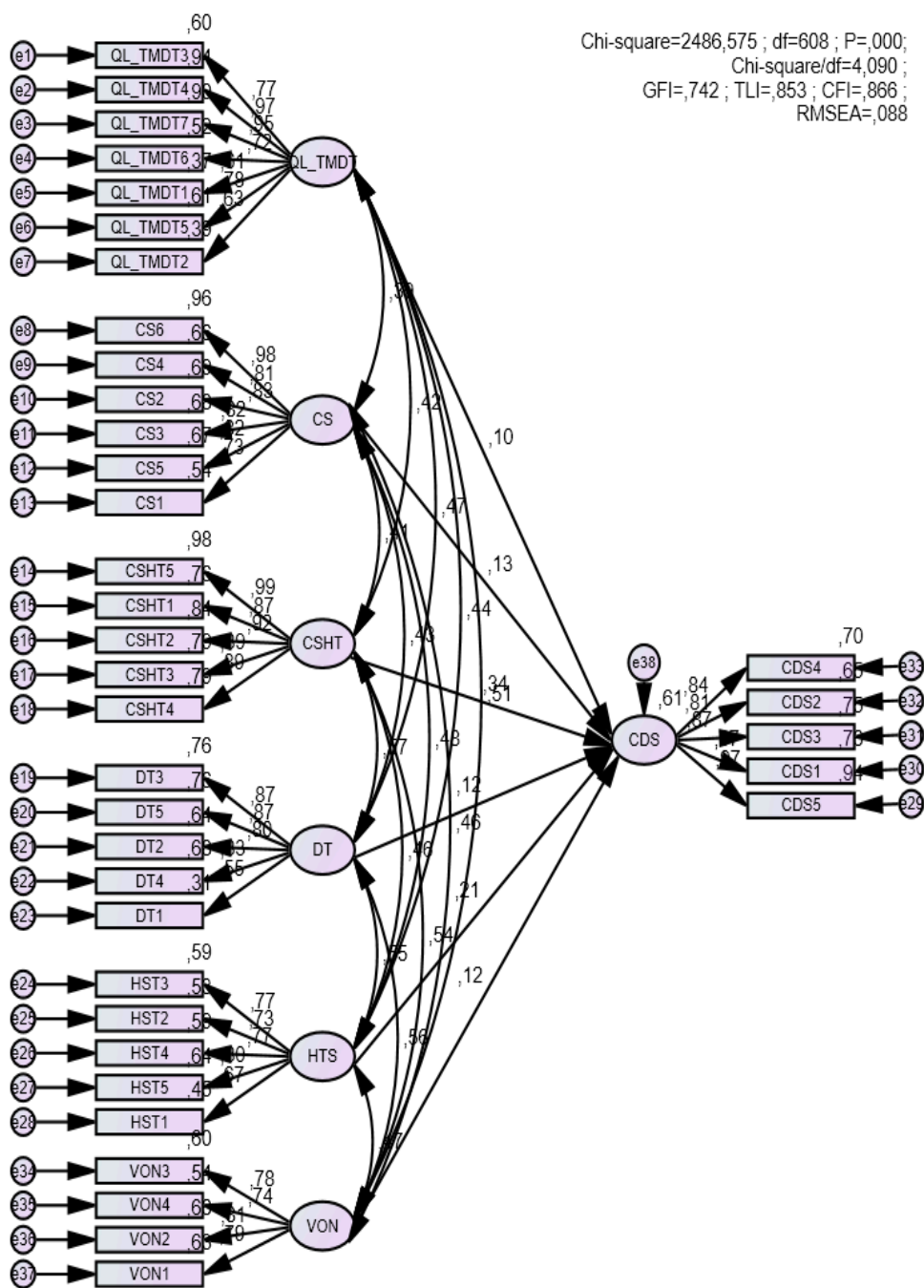
Hình 4.2. Kết quả mô hình SEM
