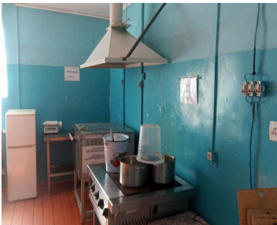
Рис.23, 24 – Местный вентотсос на кухне
