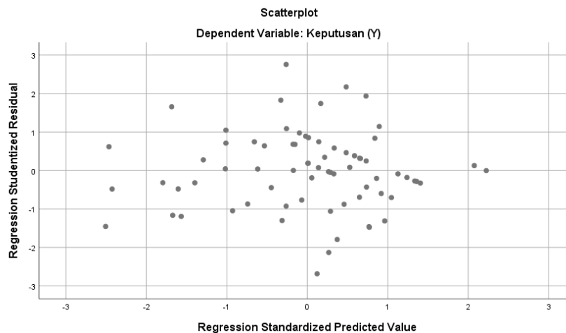
Gambar 1: Hasil uji heteroskedastisitas – grafik scatterplot
