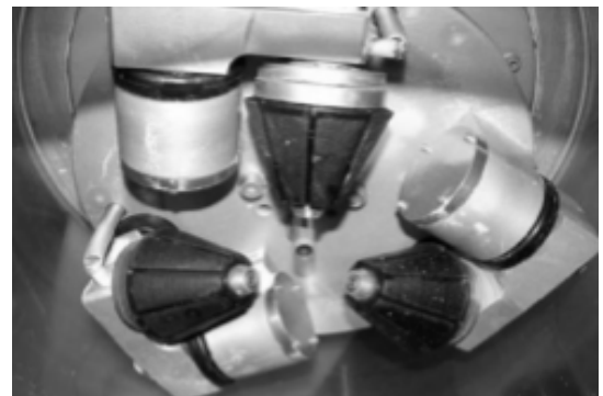
Figure 7 : tête de polissage (dessous) Tournez la page S.V.P.
