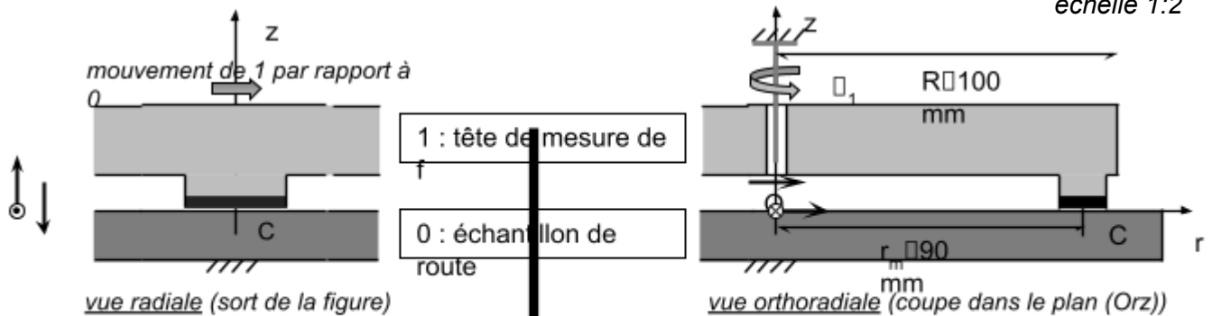
Figure D : Tête de mesure du coefficient de frottement (un seul patin est représenté)
