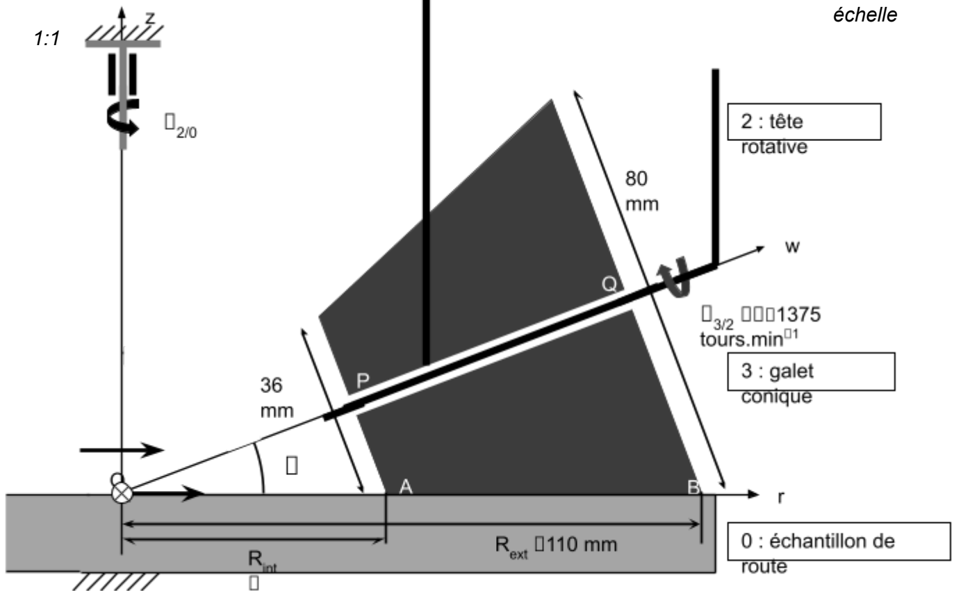
Figure E : Détail d'un galet de la tête de polissage (la tête rotative est simplement schématisée)
