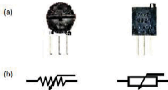
Sumber : Dokumen Kemdikbud Gambar 2.3. Resistor variabel
