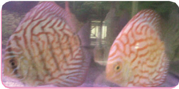
Sumber : Dokumen Kemdikbud Gambar 3.10. Discus
