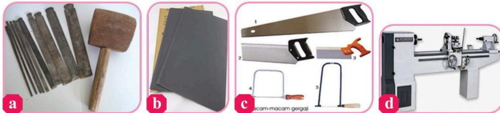
Gambar 1.29. Alat kerajinan dari kayu; a. pahat, b. amplas, c. aneka gergaji, dan d. mesin bubut.
