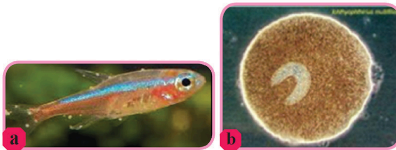
Gambar 3.38. Ikan terkena penyakit 'Ich' (a) Ichtyophthirius (b)
