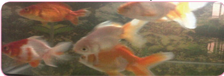
Sumber : Dokumen Kemdikbud Gambar 3.7. Jenis-jenis Koki
