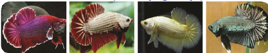
Sumber : Wikipedia.com Gambar 3.5. Cupang halfmoon
