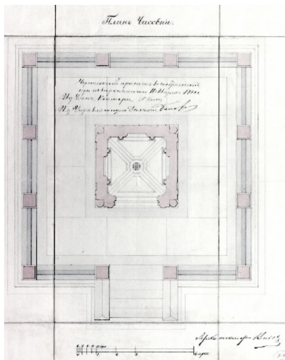
Видов А. Ф. Чертежи «План и разрез часовни». 1880. ГМЗ "Царское Село"
