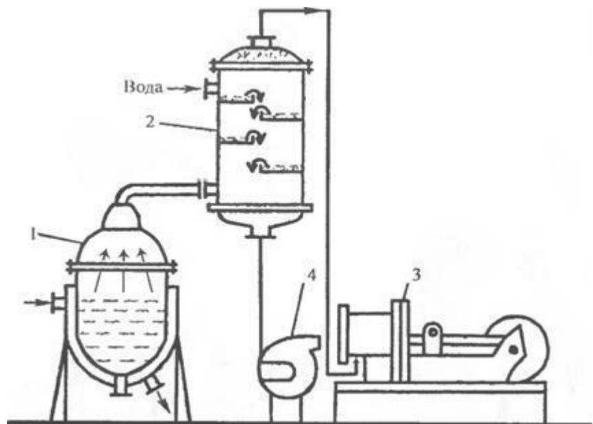
Рис. 1.2. Вакуум-випарна установка з гіротитечїйним конденсором змішування (схема Пояснення в тек
