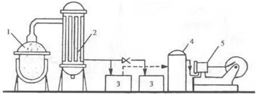
Рис. 1.1. Вакуум-випарна установка періодичної дії з поверхневим (трубчастим) конденсатором (схема). тексті
