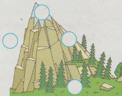
Будова гори
