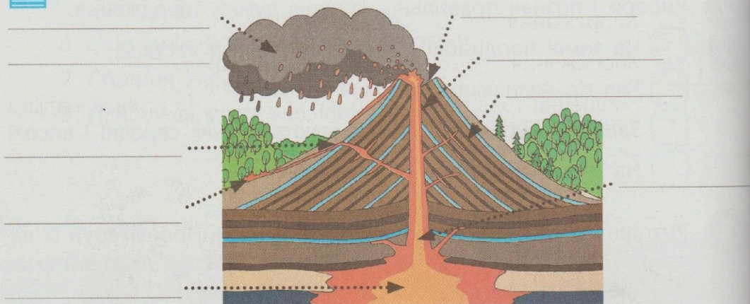
Будова вулкана
