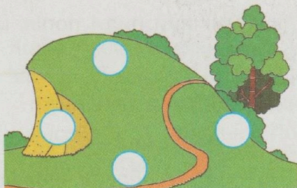
Будова горба
