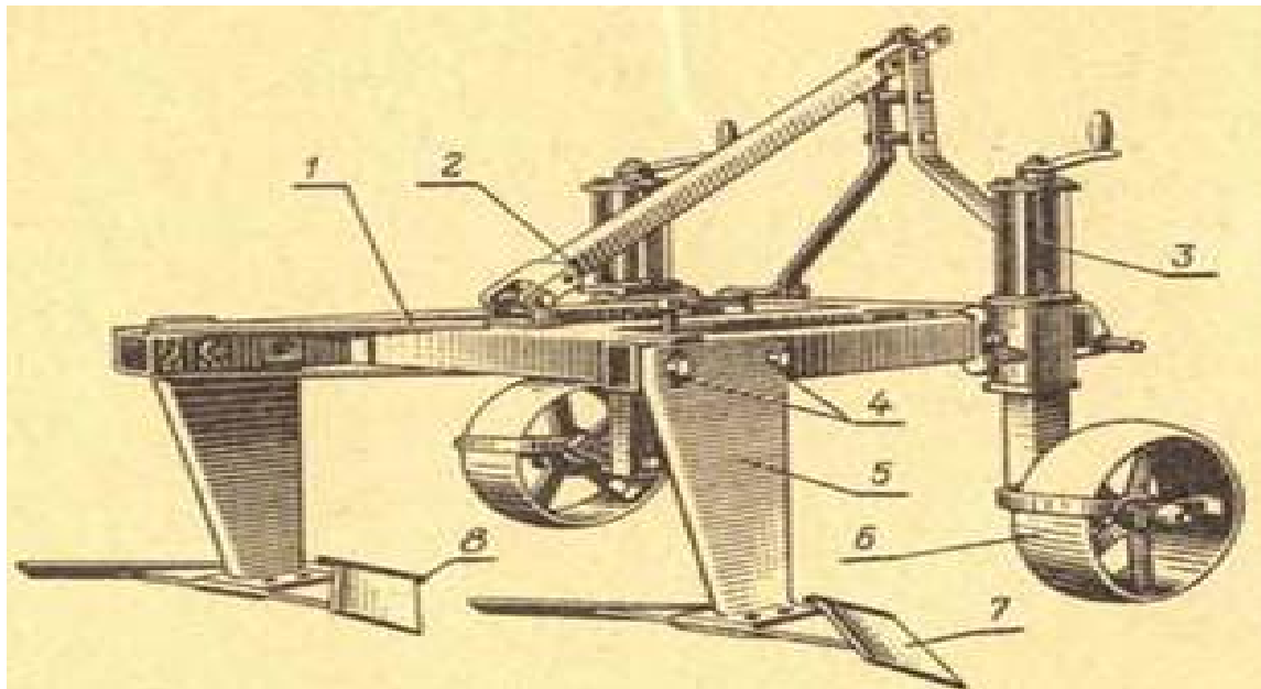
Рис. 3.3.2. Культиватор-плоскоріз КПГ-250
