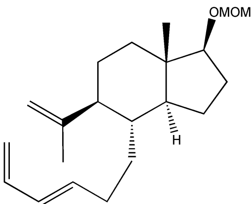
Composé W
