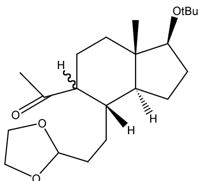
Composé R
