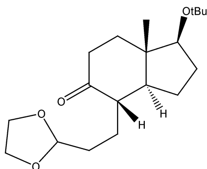
Composé N
