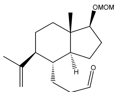
Composé U
