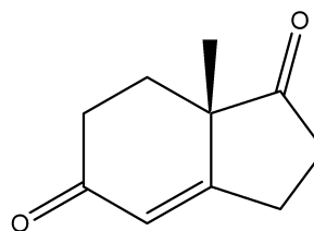
Intermédiaire A .
