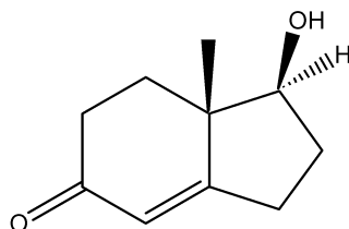
Composé I
