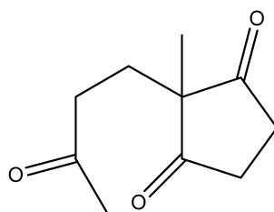
Composé F
