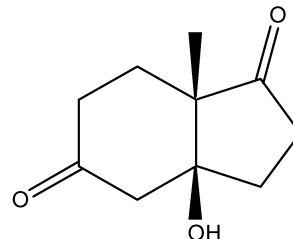
Composé G
