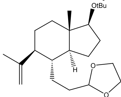
Composé T
