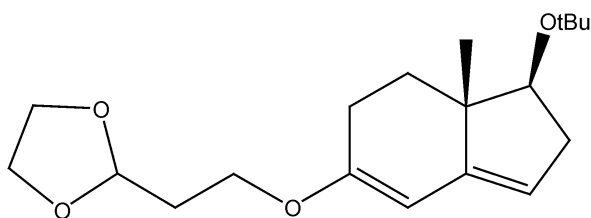
Composé K
