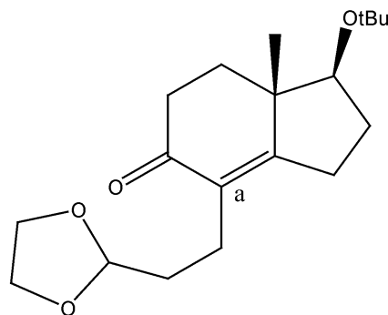
Composé L
