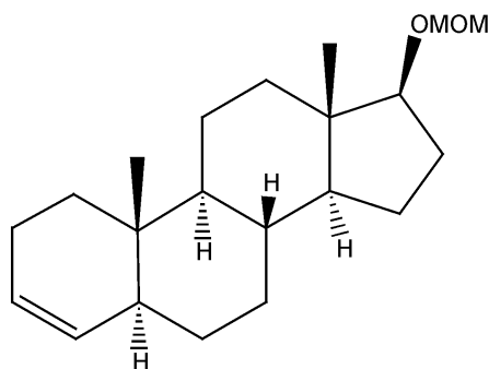
Composé X
