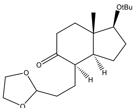
Composé M
