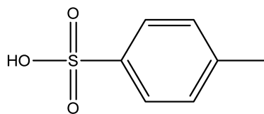
Acide paratoluènesulfonique
