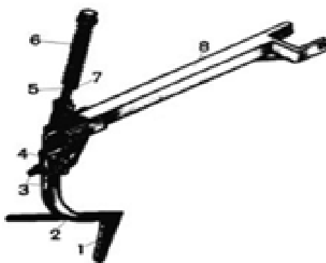
Рис.2. Будова стрільчастої лапи
