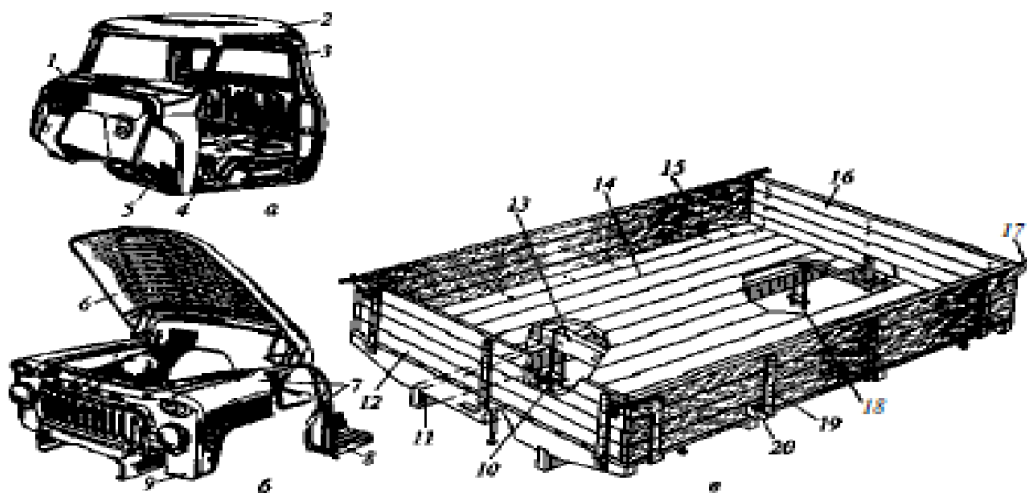
Рис. 39.9. Кузов грузового автомобиля ГАЗ.
