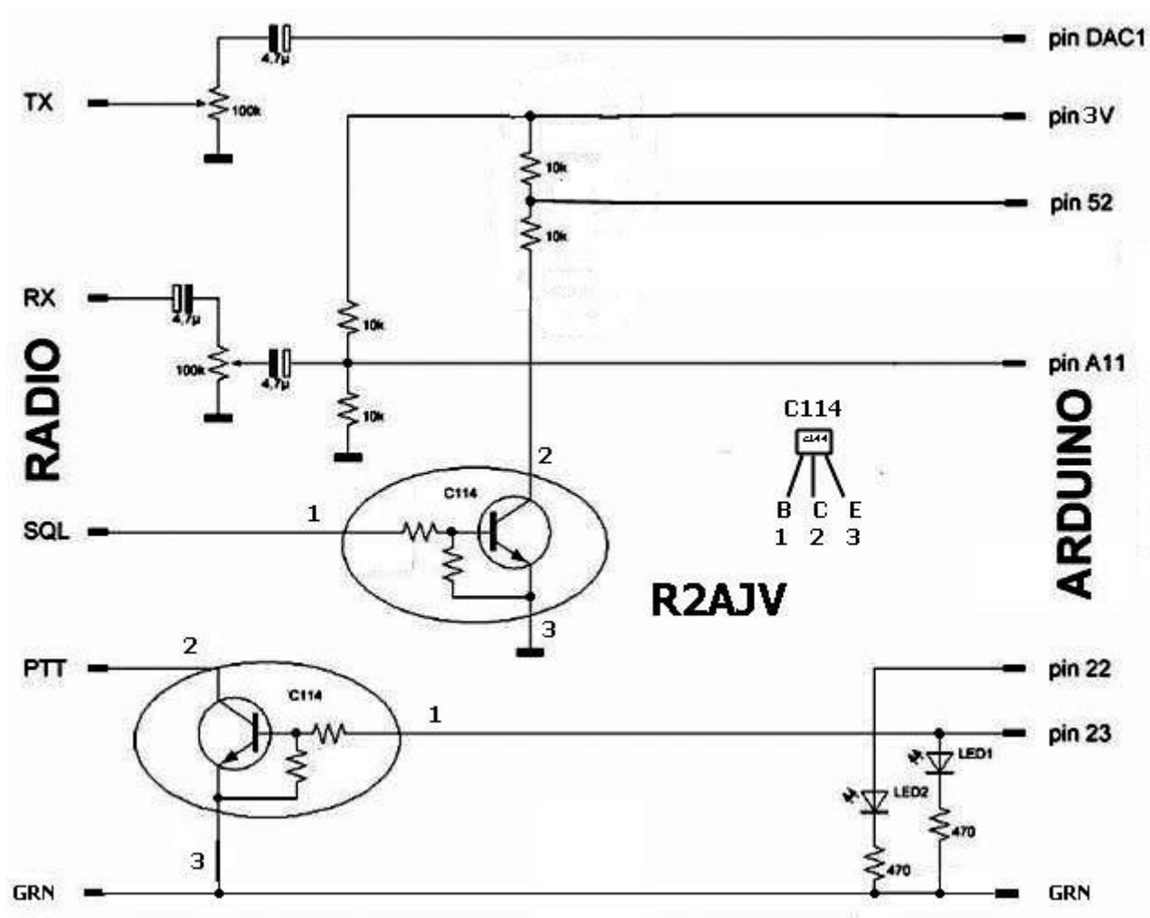
3.4.7 От UB3AIA - схема ZUM на оптопарах с линией SQL, осциллятором 14.4 и преобразованием 5v->3v
