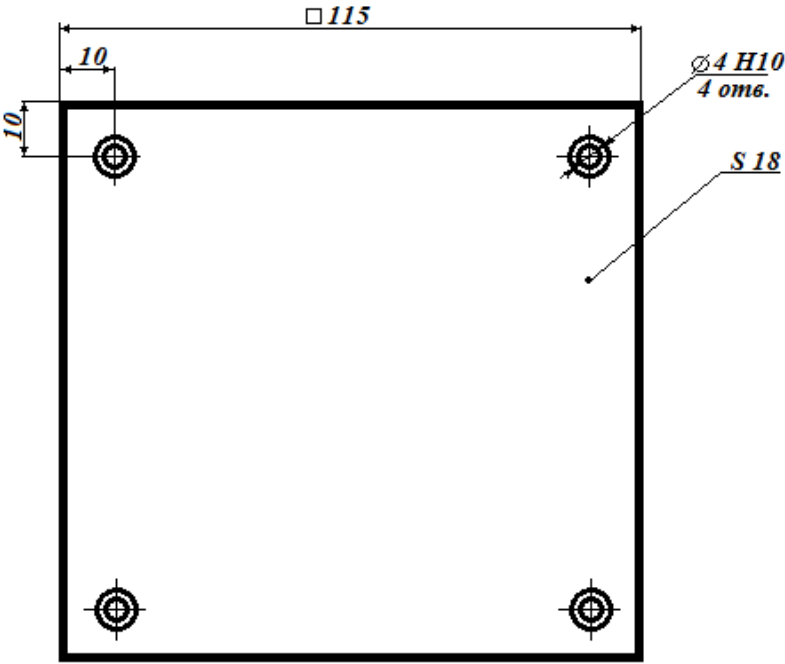
Деталь 1 (2 шт.)
