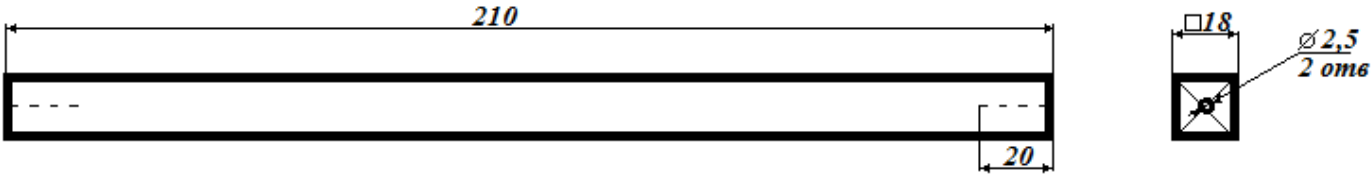
Деталь 3 (1 шт.)
