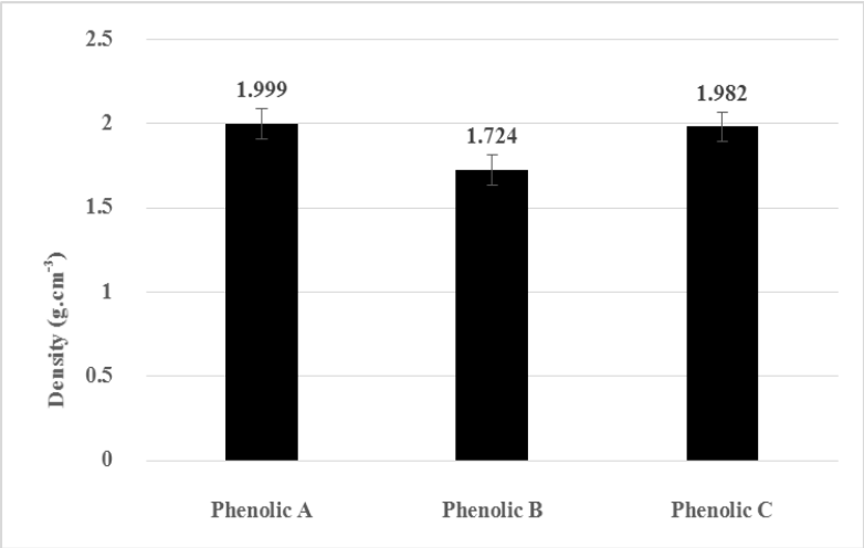
รูปที่ 2 แสดงผลของฟีนอลิก เรซินชนิด A, B และ C ตามลำดับที่เป็นองค์ประกอบในคอมโพสิตของวัสดุฉนวน ที่มีต่อค่าความหนาแน่นของวัสดุคอมโพสิต ซึ่งข้อมูลกราฟแท่งและเส้นทึบแสดงค่าเฉลี่ยของข้อมูลและความคลื่อนคลาดมาตรฐาน (จำนวนการทดลองซ้ำ เท่ากับ 3)
