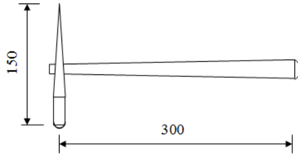
Рисунок 4.3 – Конструкція молотка Фізделя
