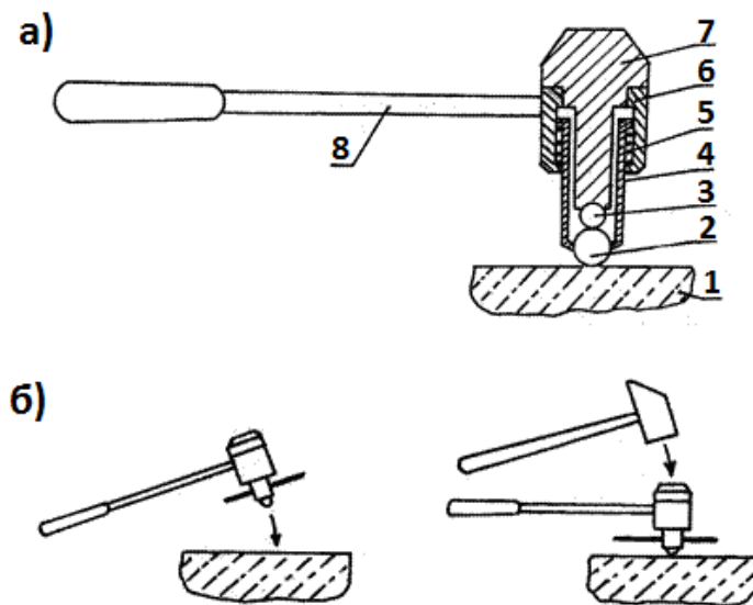
Рисунок 4.2 – Молоток Кашкарова: а – схема устрою; б – варіанти нанесення удару; 1– бетон, що випробовується; 2 – індентор (кулька); 3 – еталонний стрижень; 4 – стакан; 5 – пружина; 6 – корпус; 7 – головка; 8 – ручка
