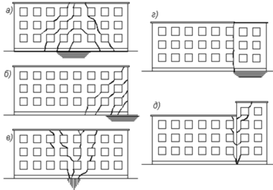
Рисунок 4.1- Розташування тріщин у цегляній кладці стін та причини їх виникнення: а – слабкий ґрунт під середньою частиною будівлі; б – те саме біля торця будівлі; в – твердий ґрунт під середньою частиною будівлі; г - просідання частини будівлі; д – різні тиски у підшві фундаментів при різнонавантажених стінах.
