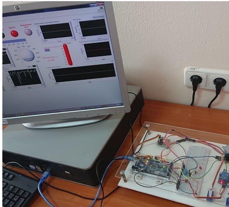
Реалізована SCADA-система
