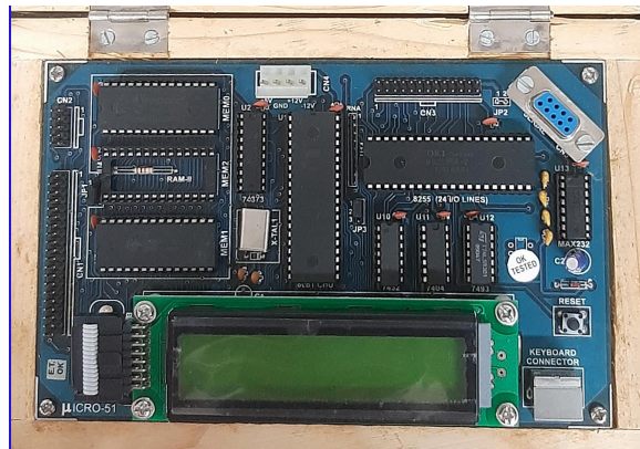
Microcontroller 8051
