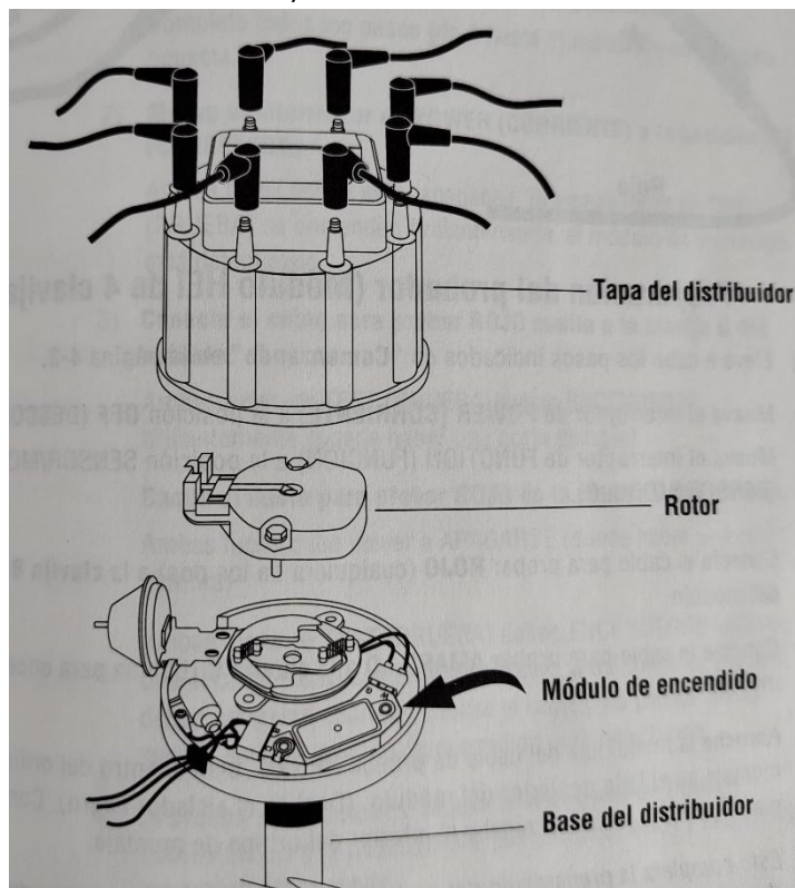
Situación típica del módulo HEI
