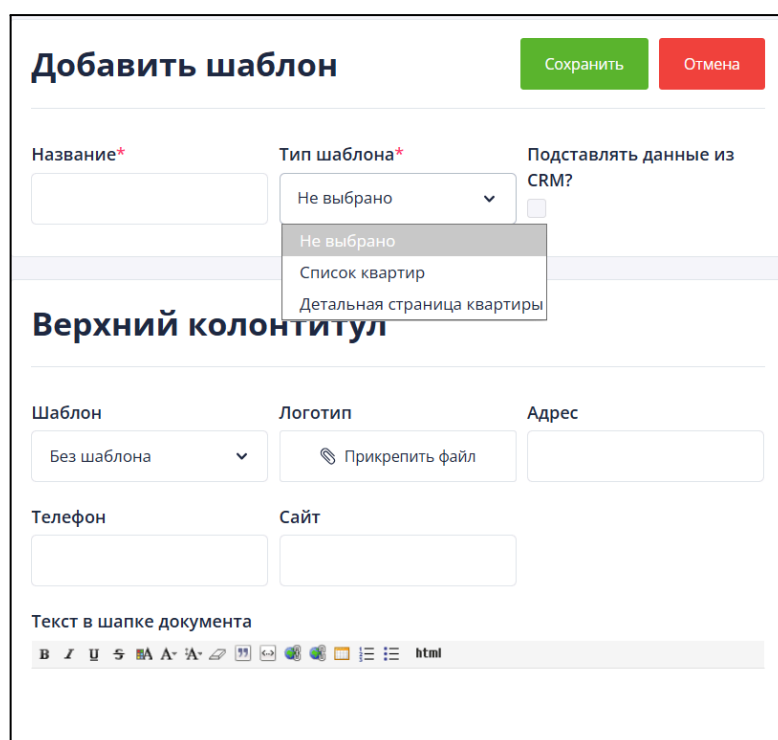
Рисунок 4.20 – Создание шаблона презентации
