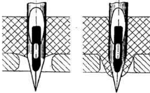
Рис. 5.1 – Прорубка трикотажного полотна голкою
