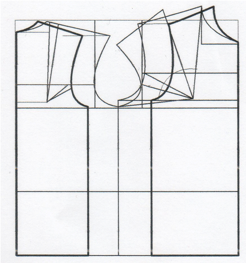
Рис. 4.2 – Проектування конструкції пілочки без нагрудної виточки
