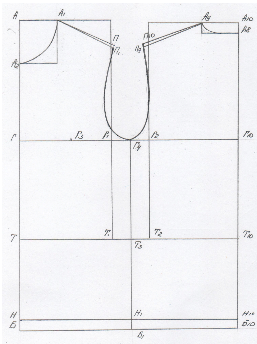
Рисунок 4.4 Побудова креслення основи плечевого жіночого одягу
