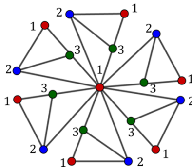
Gambar 1. Amalgamasi graf roda
