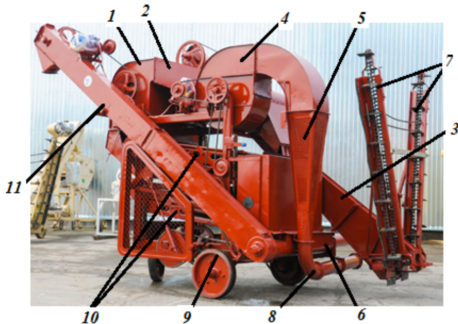
Рис. 9.1. Будова очисника вороху ОВС-25:
