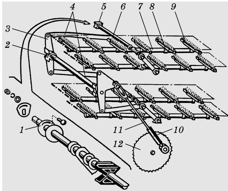
Рис. 9.2. Механізм очищення решіт ОВС -25:
