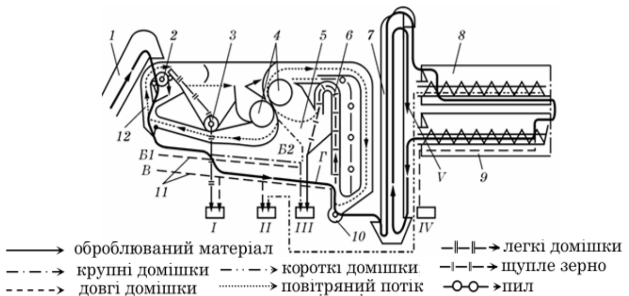
Рис. 9.5. Функціональна схема насіннеочисної машини СМ-4А:
