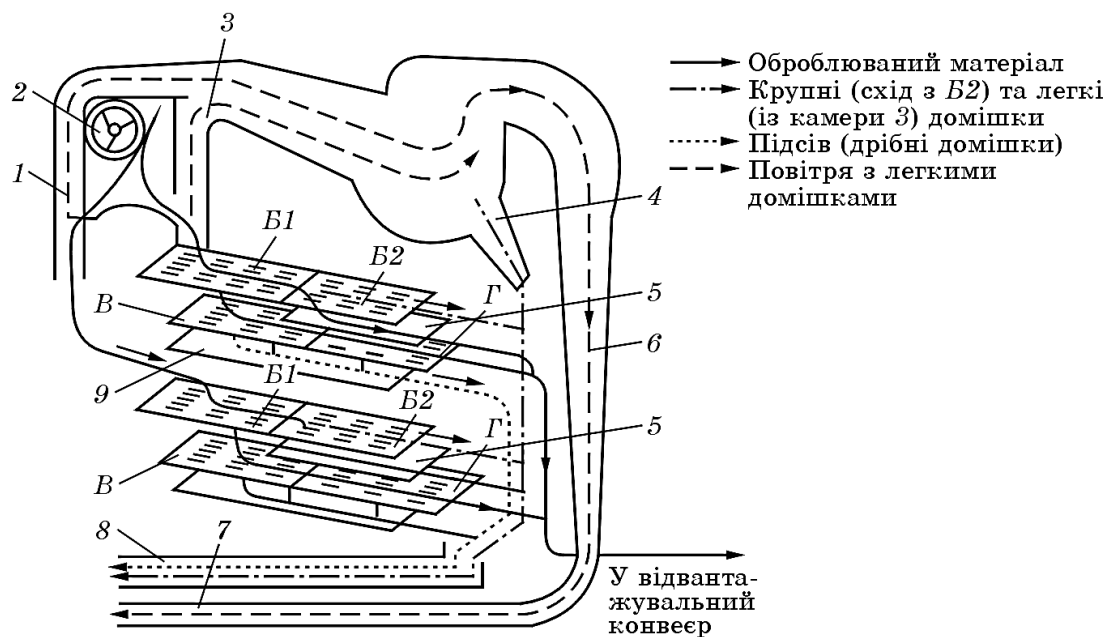
Рис. 9.3. Функціональна схема очисника вороху ОВС-25:
