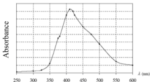
Figure 1: spectre d'absorption du dibrome gazeux
