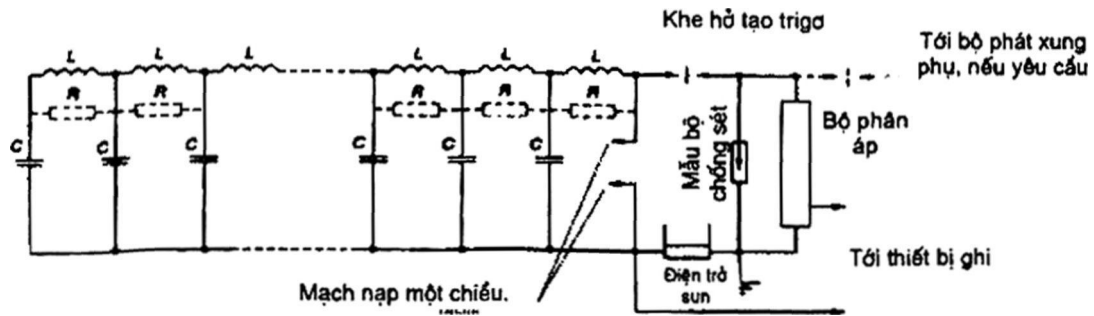
Hình D.1 - Mạch điện điển hình cho bộ phát xung phân bố không đổi cho thử nghiệm xung dòng điện thời gian dài
