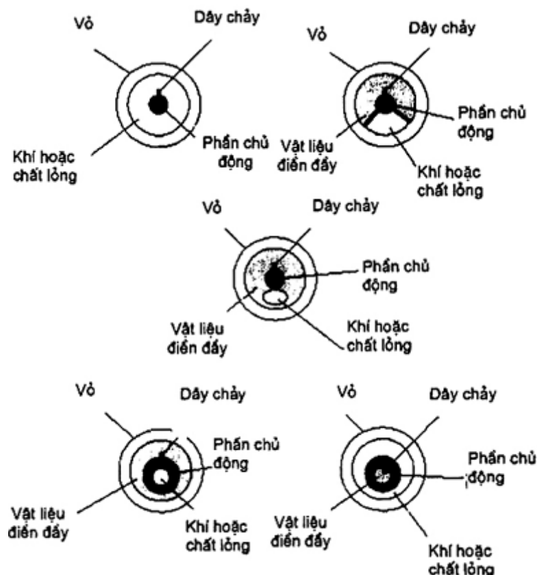
Hình 2 - Vị trí của dây chảy trong các trường hợp khác nhau
