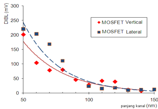
Gambar 1. Tren DIBL untuk MOSFET (Bold, Cambria 10pt)
