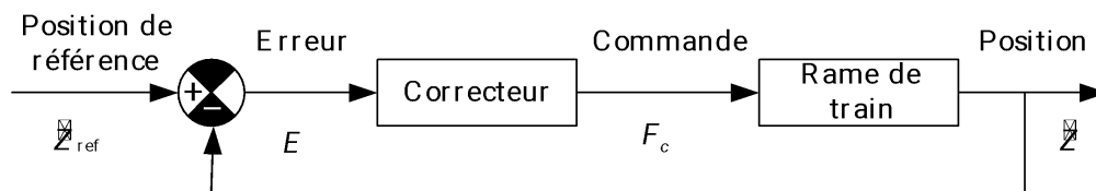
Figure 5 : Système d'asservissement de la position verticale d'une rame de train E.D.S..
