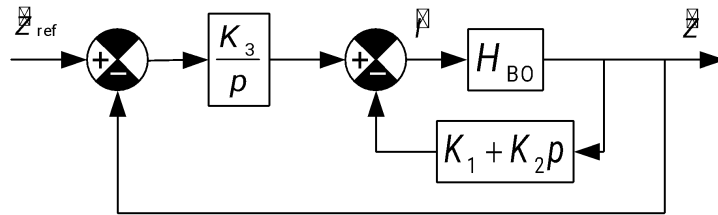
Figure 9 : Nouveau schéma de commande.
