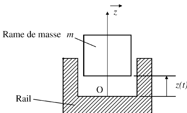
Figure 4 : Modélisation élémentaire de la rame.
