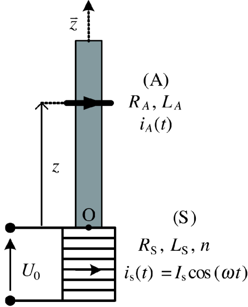
Figure 2 : Une réalisation de l'expérience d'Élihu Thomson.
