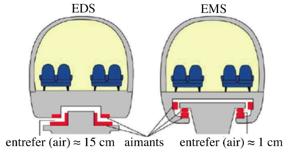
Figure 3 : Technologies EDS (répulsion) et EMS (attraction) de trains à lévitation magnétique.
