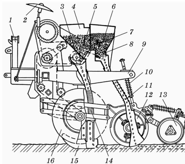
Рис . 5.10. Функціональна схема овочевої сівалки СО -4,2:
