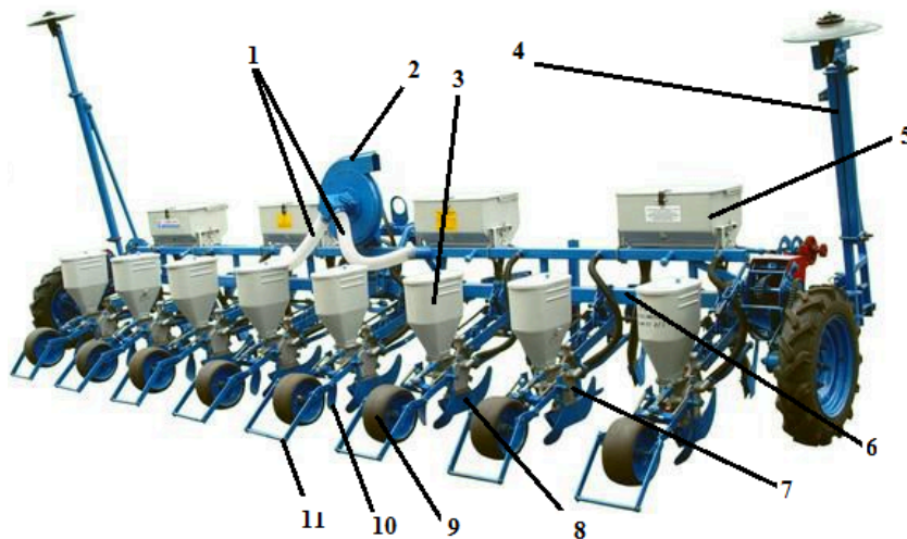
Рис. 5.1. Універсальна пневматична сівалка СУПН-8А:
