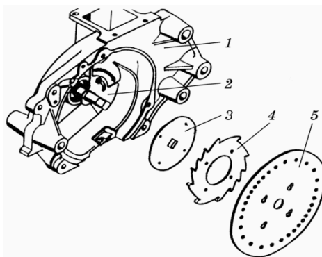
Рис . 5.4. Висівний апарат сівалки УПС -12:
