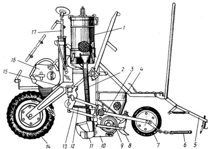
Рис.4. Будова сівалки ССТ-12Б
