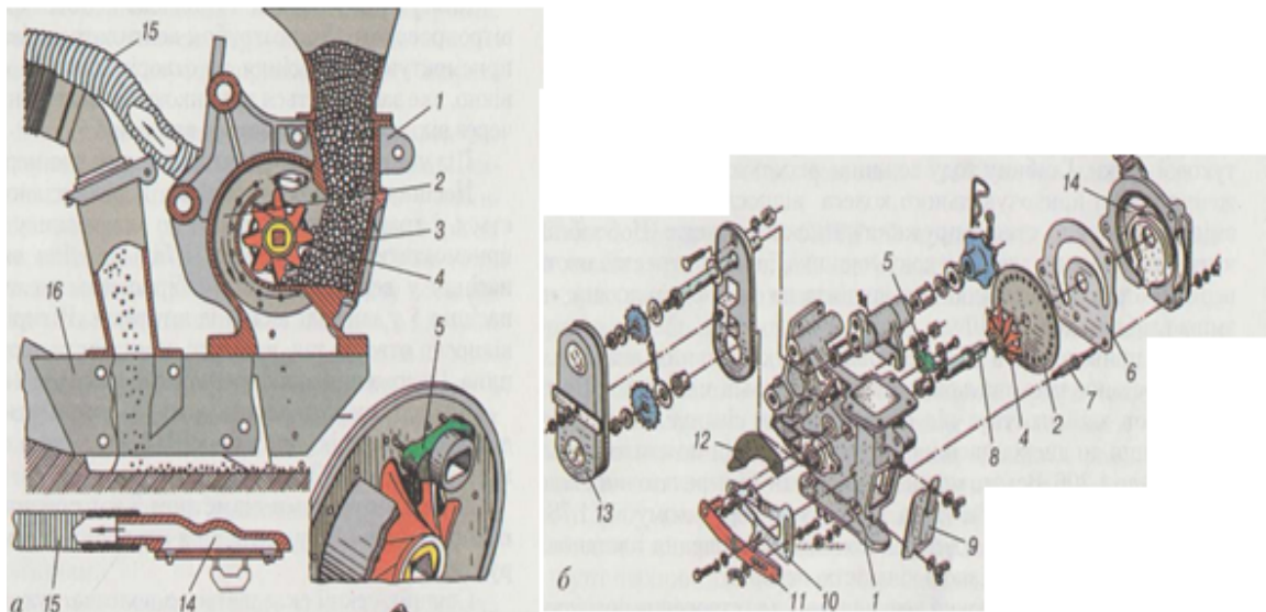
Рис. 5.2. Дисківий пневматичний висівний апарат сівалки СУПН-8А:
