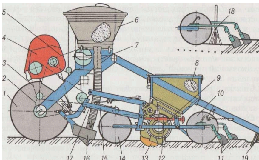
Рис. 5.6. Схема технологічного процесу роботи сівалки ССТ-12В:
