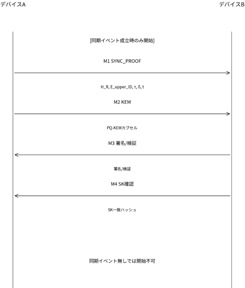
図9 プロトコル時系列（同期トリガ）
