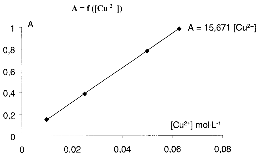
Figure 1 : Absorbance mesurée à \lambda_{\max} = 811 \text{ nm} à 25^\circ\text{C} dans une solution d'acide nitrique.
