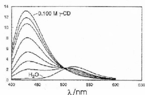
FIG. 21 – Spectres d'émission de fluorescence d'une solution de PRODAN dans une solution aqueuse contenant, par ordre d'intensité croissante, 0 ; 0,007 ; 0,010 ; 0,015 ; 0,025 ; 0,050 ; 0,070 ; 0,100 mol.L -1 de γ-Cy-D. L'intensité de fluorescence est donnée en fonction de la longueur d'onde du rayonnement réémis (en nm).
