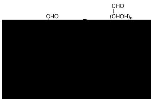
FIG. 3 – Nomenclature D ou L des sucres
