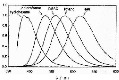
FIG. 20 – Spectres d'émission de fluorescence de solutions de PRODAN à 10^{-6} mol.L -1 dans différents solvants. L'intensité de fluorescence est tracée en fonction de la longueur d'onde du rayonnement réémis (en nm).
