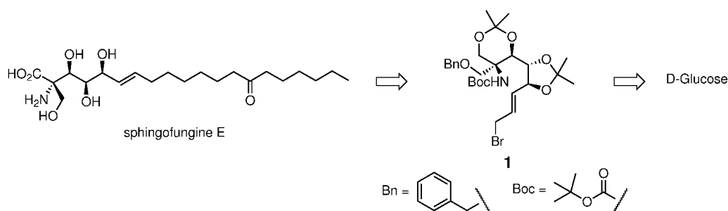
FIG. 14 – Rétrosynthèse de la Sphingofungine E
