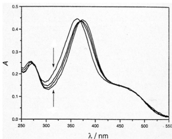
FIG. 25 – Spectres d'absorption UV-visible pour le substrat S en solution aqueuse. Les solutions contiennent, en lisant de haut en bas au niveau des flèches : [S]_0 = 3,338 \cdot 10^{-5} \text{ mol.L}^{-1} (identique pour toutes les solutions) ; [C]_0 = 0 ; 8,350 \cdot 10^{-4} ; 3,340 \cdot 10^{-3} ; 6,680 \cdot 10^{-3} \text{ mol.L}^{-1}
