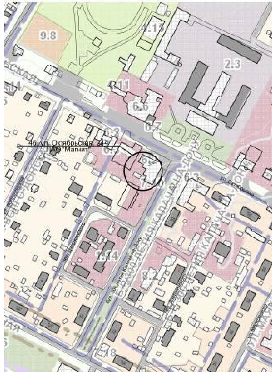
Схема размещения места (площадки) накопления ТКО на территории Калачевского городского поселения М 1:2000 46. г. Калачин-Дону, ул. Октябрьская, 244 ПАО "Магнит"
