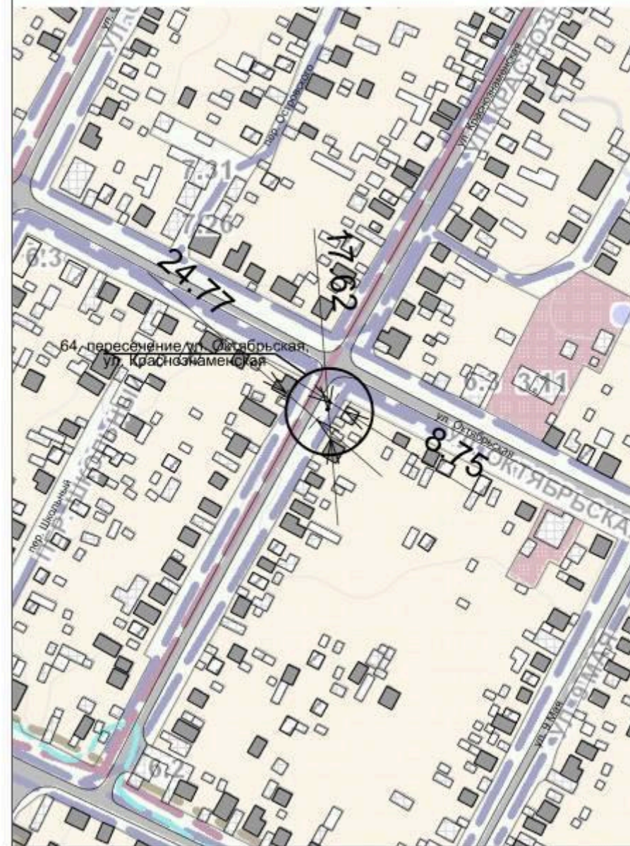
Схема размещения места (площадки) накопления ТКО на территории Калачевского городского поселения М 1:2000 64. г. Калач-на-Дону, пересечение ул. Октябрьская, ул. Краснознаменная
