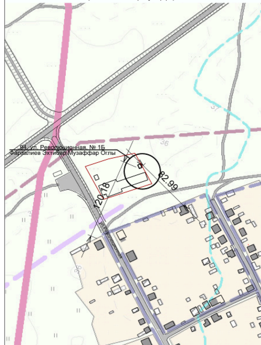
Схема размещения места (площадки) накопления ТКО на территории Калачевского городского поселения М 1:2000 94. г. Калач-на-Дону, ул. Революционная, №1Б Фарзалиев Эхтибар Музаффар Оглы
